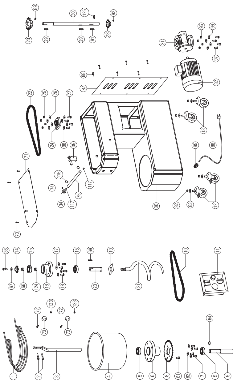
FIG. 18 Parti di ricambio impastatrice con testa e vasca fissa mod. IM 12-18 FIG. 18 Pièces de rechange pour pétrisseuse avec tête et cuve fixe mod. IM 12-18 PICT. 18 Spare parts for mixer with fixed top and bowl mod. IM 12-18 BILD 18 Ersatzteile für die Teigknetmaschine mit gestemt Kopf und Becken mod. IM 12-18
