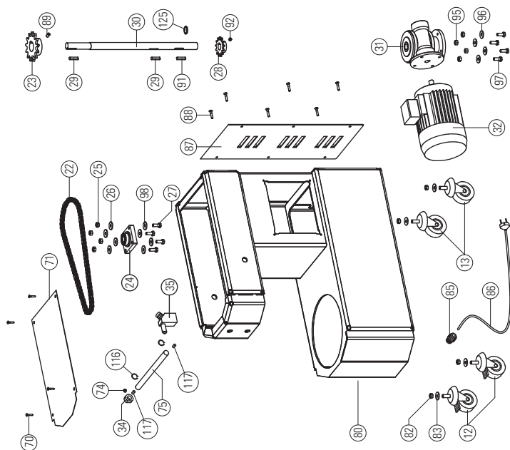
BILD 19 Ersatzteile für die Teignetmaschine mit gestern Kopf und Becken mod. IM 25-38-44
