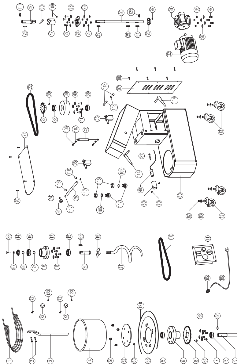
FIG. 21 Parti di ricambio impastatrice con testa sollevabile e vasca estraibile mod. IM 12-18 A FIG. 21 Pièces de rechange pour pétrisseuse avec tête soulevable et cuve extractible mod. IM 12-18 A PICT. 21 Spare parts for mixer with raising top and removable bowl mod. IM 12-18 A BILD 21 Ersatzteile für die Teigknetmaschine mit hebbarem Kopf und herausziehbarem Becken mod. IM 12-18 A
