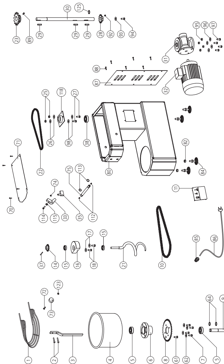
PICT. 17 Spare parts for mixer with fixed top and bowl mod. IM 5-8 BILD 17 Ersatzteile für die Teigknetmaschine mit gestern Kopf und Becken mod. IM 5-8
