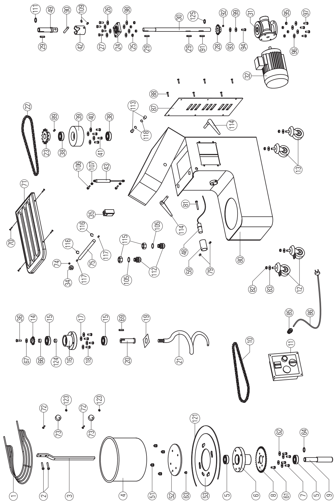
FIG. 21 Parti di ricambio impastatrice con testa sollevabile e vasca estraibile mod. PK 12-18 A FIG. 21 Pièces de rechange pour pétrisseuse avec tête soulevable et cuve extractible mod. PK 12-18 A PICT. 21 Spare parts for mixer with raising top and removable bowl mod. PK 12-18 A BILD 21 Ersatzteile für die Teignet-maschine mit hebbaarem Kopf und herausziehbarem Becken mod. PK 12-18 A
