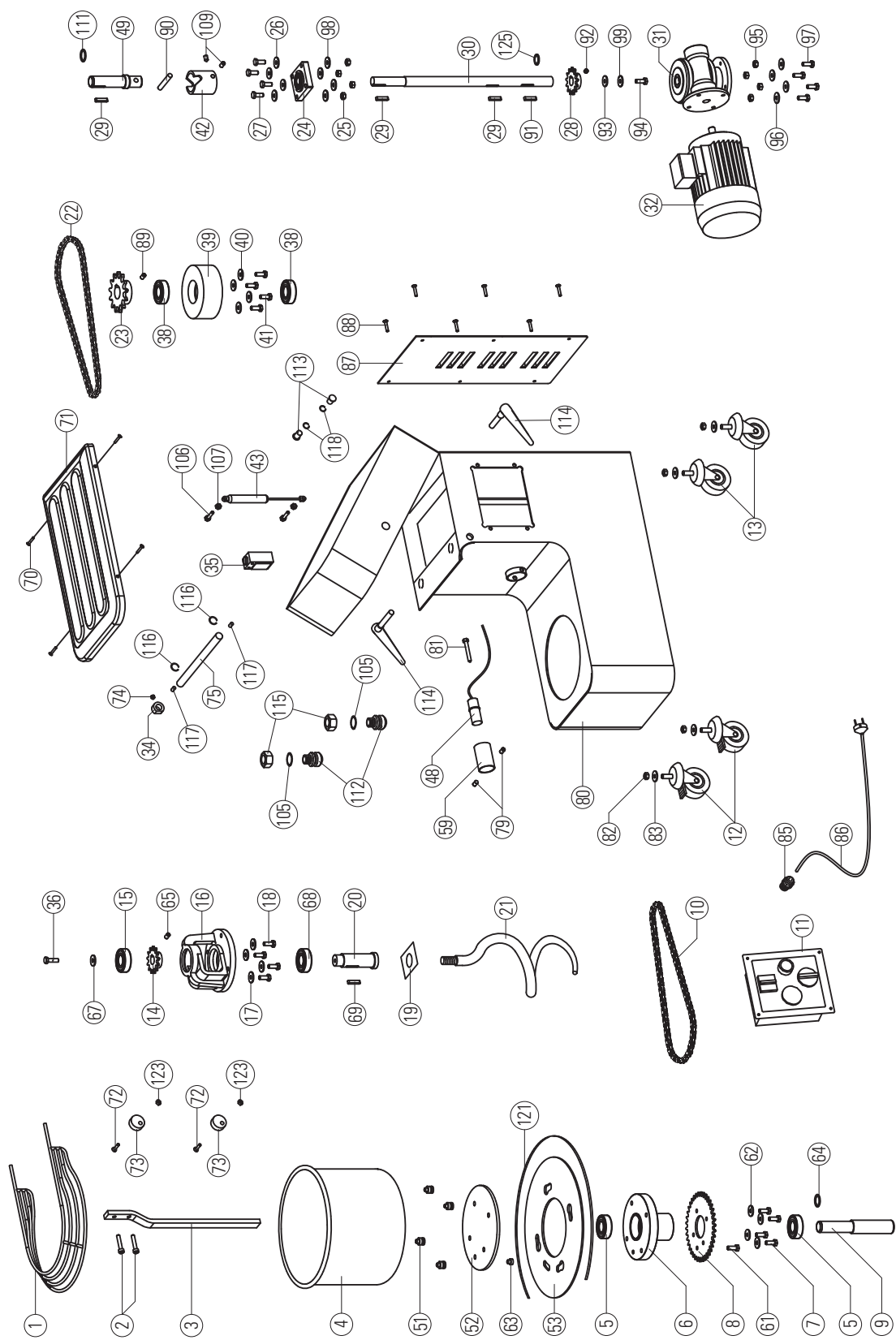
FIG. 22 Parti di ricambio impastatrice con testa sollevabile e vassa estraibile mod. PK 25-38-44 A
